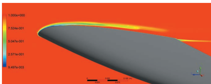
Rys. 10. Intermitencja w warstwie przyściennej ukazująca przejście warstwy laminarnej w turbulentną
